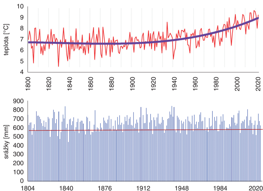
Obr. 3: Průběh průměrných ročních teplot (nahore) a úhrnů ročních srážek s vyznačením průměru (dole) na území České republiky v uvedeném období Zdroj: Údaje Czech-Globe poskytl k využití prof. Ing. Zdeněk Žalud, Ph.D. [10]
